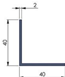
L40x40
